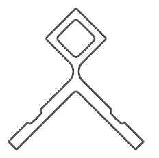
Bordure de coin extérieur UH51 75 x 77.5 mm (3.0 x 3.1 po)
