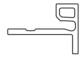
Bordure de finition UH50 75 x 54 mm (3.0 x 2.1 po)
